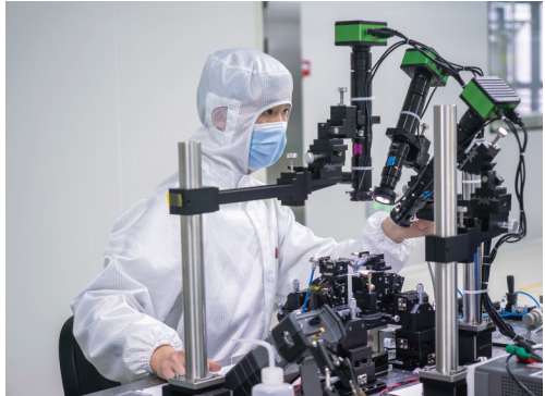
国盾量子光电混合集成器件微组装生产线
