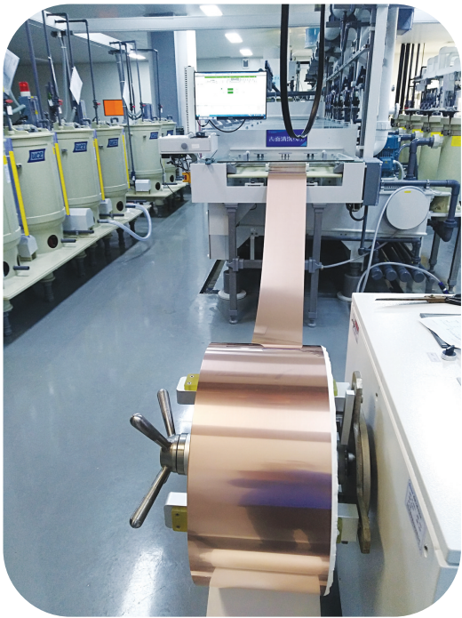
新恒汇电子科技有限公司引线框架表面清洗线
